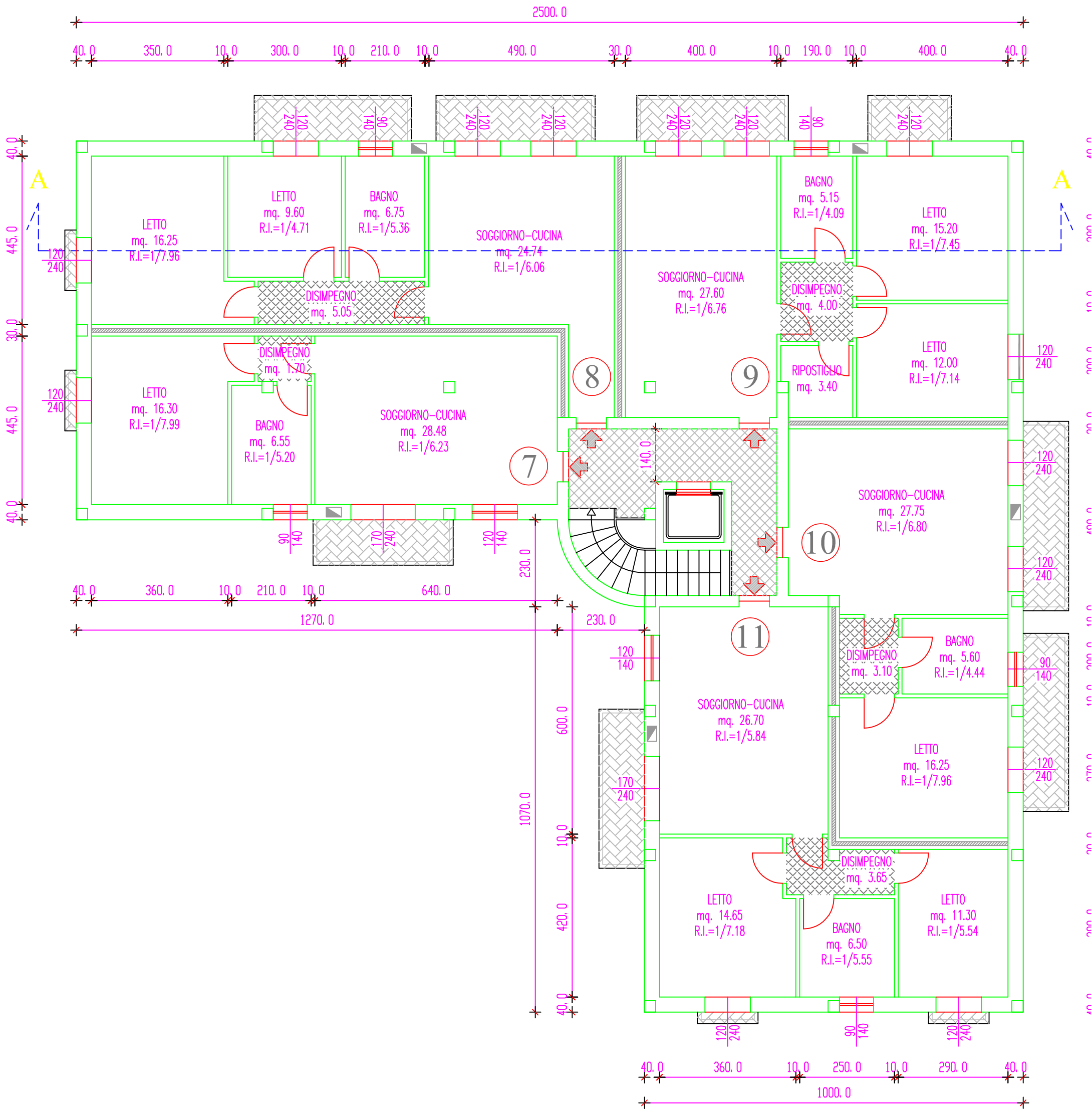
PIANTA PIANO SECONDO
